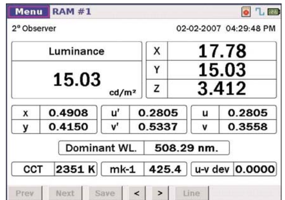
タッチパネル画面への測定結果表示例
